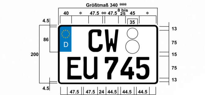
Zweizeiliges Europa-Kennzeichen FE-Mittelschrift
