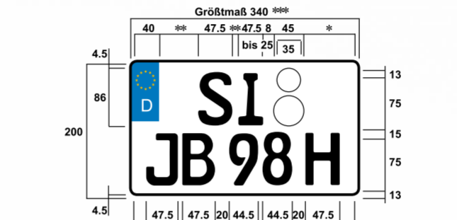
Zweizeiliges Oldtimer-Kennzeichen FE-Mittelschrift
