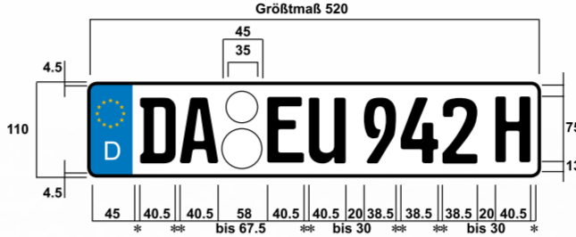
Einzeiliges Oldtimer-Kennzeichen FE-Engschrift, * Mindestmaß 8 mm ** 8 - 10 mm
