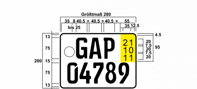
Zweizeiliges Kurzzeit-Kennzeichen FE-Engschrift, * Mindestmaß 8 mm ** 8 - 10 mm *** Bei zwei- und dreistelligen Kfz 280 mm
