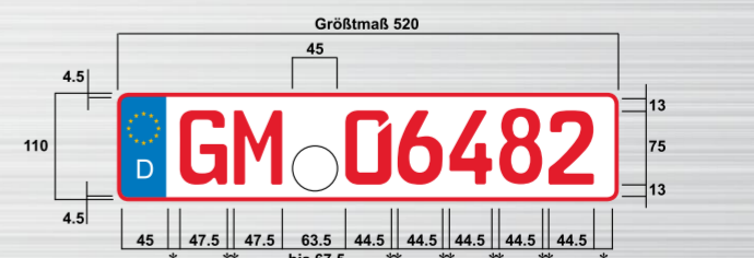
Einzeiliges Kennzeichen für Händler FE-Mittelschrift, * Mindestmaß 8 mm ** 8 - 10 mm
