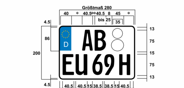
Zweizeiliges Oldtimer-Kennzeichen FE-Engschrift, * Mindestmaß 8 mm ** 8 - 10 mm *** Bei zwei- und dreistelligen Kfz 280 mm oder **** 15 - 30 mm Zur Herstellung eines kürzeren Kennzeichen Plaketten unter dem Euro-Feld anbringen.
