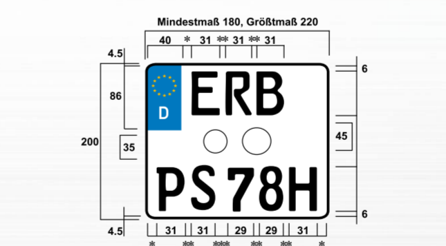
Kraftrad-Kennzeichen FE-Schrift 49 mm, (Kraftrad-Kennzeichen) * Mindestmaß 8 mm ** 8 - 10 mm *** 15 - 18 mm
