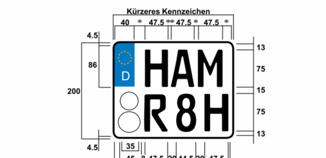
Zweizeiliges Oldtimer-Kennzeichen, verkürzt FE-Mittelschrift, * Mindestmaß 8 mm ** 8 - 10 mm *** Bei zwei- und dreistelligen Kfz 280 mm
