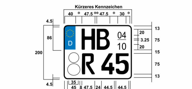
Zweizeiliges Saison-Kennzeichen, verkürzt FE-Mittelschrift, * Mindestmaß 8 mm ** 8 - 10 mm *** Bei zwei- und dreistelligen Kfz 280 mm
