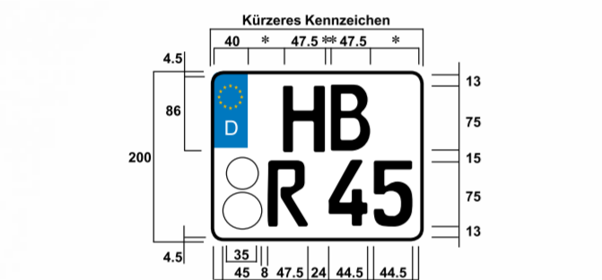
Zweizeiliges Europa-Kennzeichen, verkürzt FE-Mittelschrift, * Mindestmaß 8 mm ** 8 - 10 mm *** Bei zwei- und dreistelligen Kfz 280 mm
