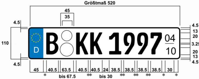
Einzeiliges Saison-Kennzeichen FE-Engschrift, * Mindestmaß 8 mm ** 8 - 10 mm
