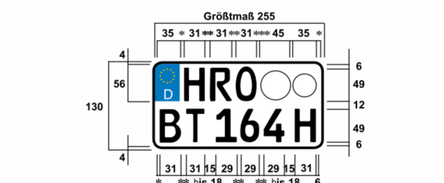
Zweizeiliges Oldtimer-Kennzeichen, verkleinert FE-Schrift 49 mm, (Leichtkrafträder und Zugmaschinen) * Mindestmaß 6 mm ** 8 - 10 mm *** 5 - 20 mm
