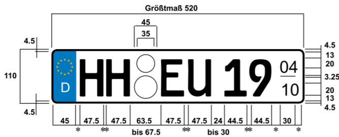
Einzeiliges Saison-Kennzeichen FE-Mittelschrift
