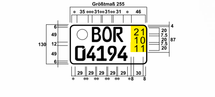
Zweizeiliges Kurzzeit-Kennzeichen, verkleinert FE-Schrift 49 mm, (Leichtkrafträder und Zugmaschinen) * Mindestmaß 6 mm ** 8 - 10 mm *** 5 - 20 mm
