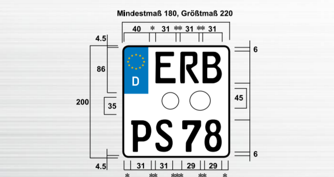
Kraftrad-Kennzeichen FE-Schrift 49 mm, (Kraftrad-Kennzeichen) * Mindestmaß 8 mm ** 8 - 10 mm *** 15 - 18 mm
