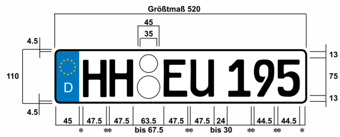
Einzeiliges Europa-Kennzeichen FE-Mittelschrift
