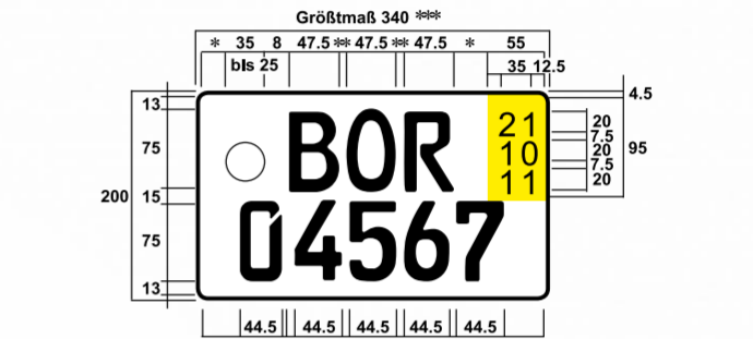
Zweizeiliges Kurzzeit-Kennzeichen FE-Mittelschrift
