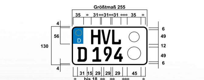
Zweizeiliges Europa-Kennzeichen, verkleinert FE-Schrift 49 mm, (Leichtkrafträder und Zugmaschinen) * Mindestmaß 8 mm ** 8 - 10 mm *** 5 - 20 mm
