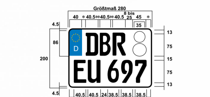
Zweizeiliges Europa-Kennzeichen FE-Engschrift
