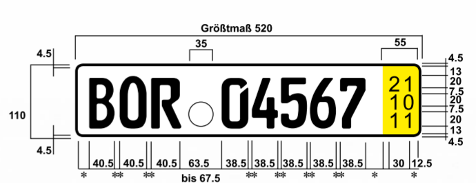
Einzeiliges Kurzzeit-Kennzeichen FE-Engschrift, * Mindestmaß 8 mm ** 8 - 10 mm
