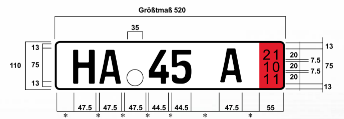
Einzeiliges Ausfuhr-Kennzeichen FE-Mittelschrift, * Mindestmaß 8 mm ** 8 - 10 mm
