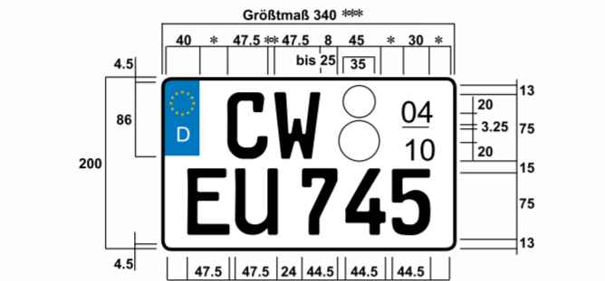
Zweizeiliges Saison-Kennzeichen FE-Mittelschrift
