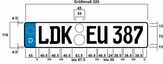
Einzeiliges Europa-Kennzeichen FE-Engschrift, * Mindestmaß 8 mm ** 8 - 10 mm
