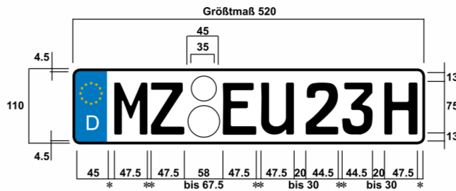
Einzeiliges Oldtimer-Kennzeichen FE-Mittelschrift
